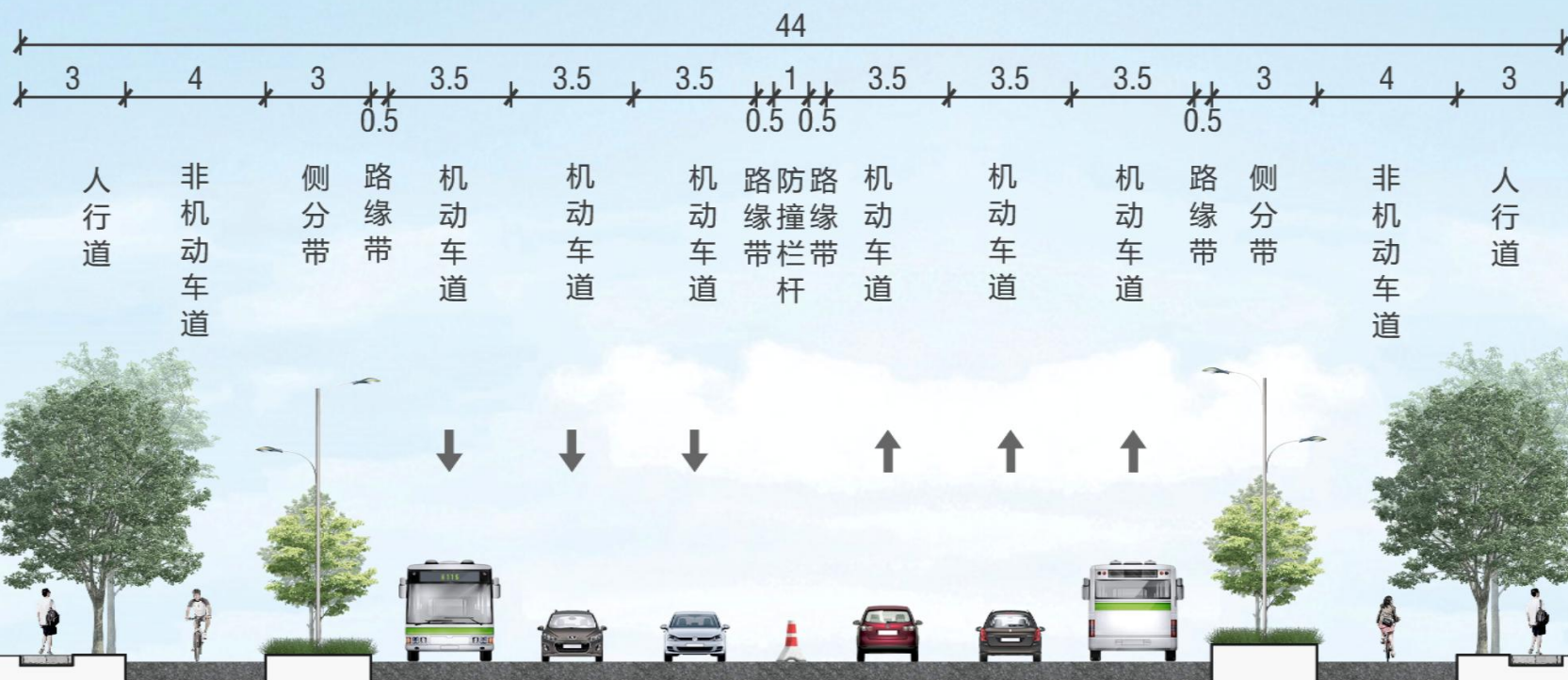
鲁肃大道标准横断面图(44m)-推荐方案
