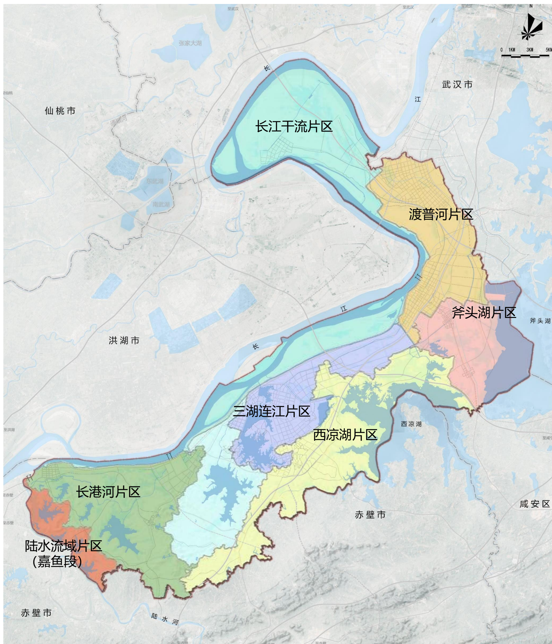
嘉鱼县四级流域分片图
